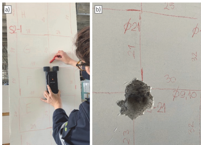
Slika 8. a) Lociranje armature, određivanje debljine zaštitnog sloja i promjera armature uređajem zasnovanim na vrtložnim strujama; b) Potvrđivanje lokacije otvaranjem zaštitnog sloja betona [19]
