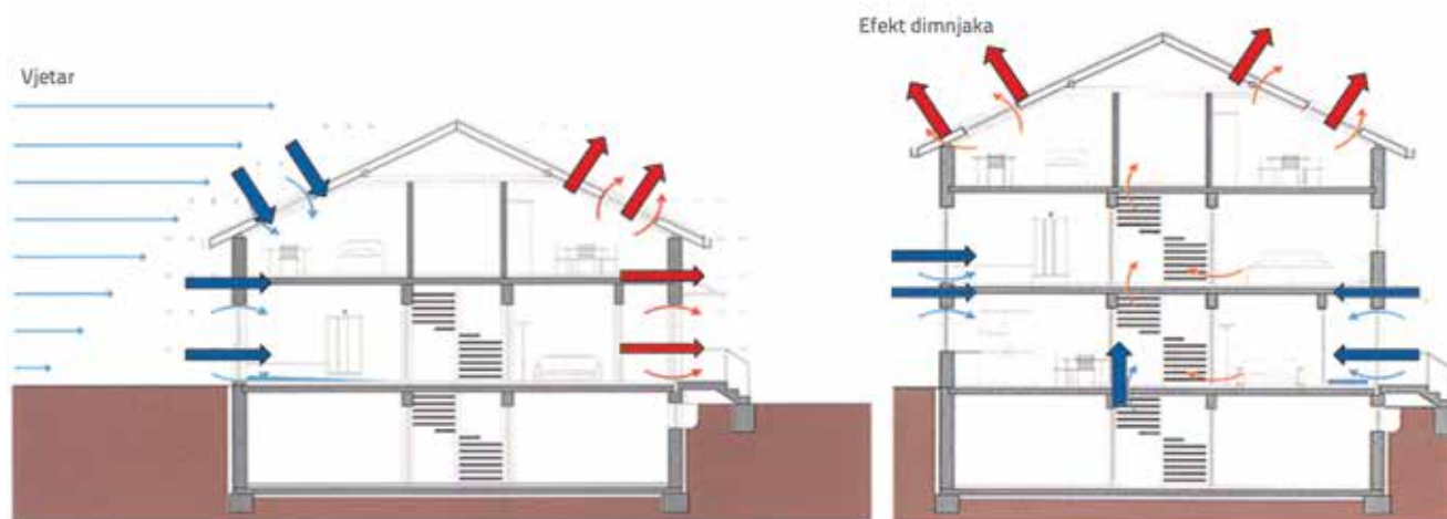
Slika 6. Shematski prikaz infiltracije i eksfiltracije zraka kroz građevne dijelove zgrade
