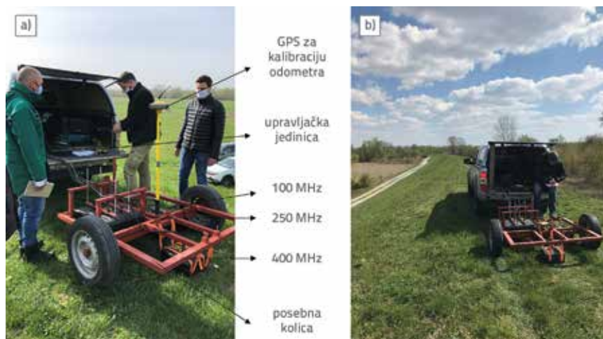
Slika 14. Ispitivanje oštećenja savskih i uspornih nasipa u gradu Zagrebu i okolici nakon potresa u ožujku 2020.: a) prikaz opreme za prikupljanje podataka, b) provedba prikupljanja podataka
