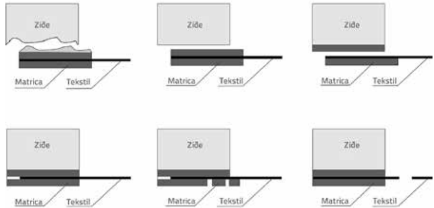
Slika 4. Modovi otkazivanja [25]
