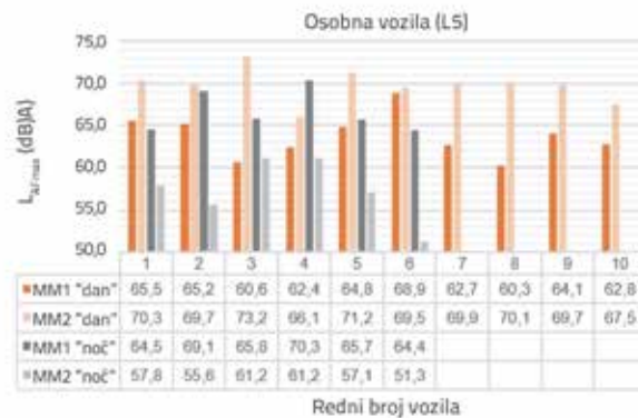
Slika 16. Rezultati mjerenja buke pojedinačnih vozila na lokaciji L5
