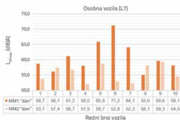
Slika 18. Rezultati mjerenja buke pojedinačnih vozila na lokaciji L7
