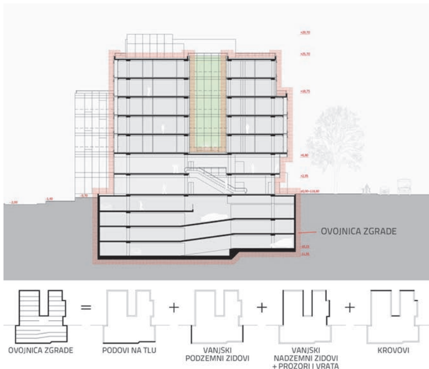
Slika 3. Ovojnice zgrade
