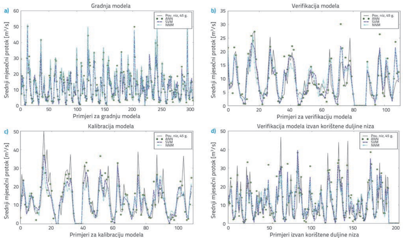
Slika 7. Primjeri uz drugi pristup: a) Izgradnja; b) kalibracija; c) verifikacija; d) verifikacija izvan korištene duljine niza modela za povijesni niz duljine 45 godina
