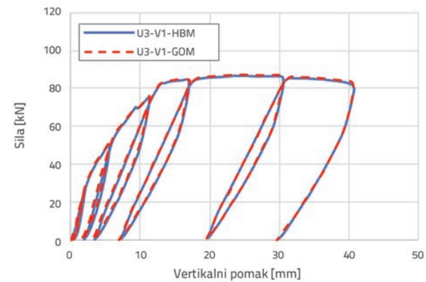
Slika 14. Usporedba dijagrama sila-pomak za uzorak U3
