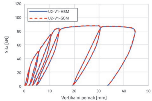
Slika 12. Usporedba dijagrama sila-pomak za uzorak U2
