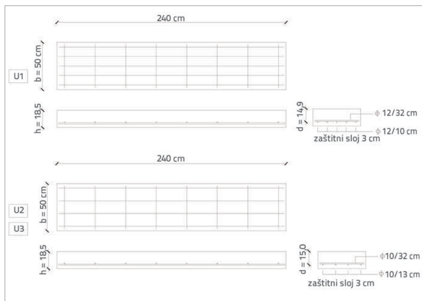
Slika 4. Plan armature
