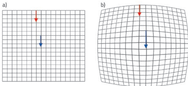
Slika 1. Distorzija leće fotoaparata
