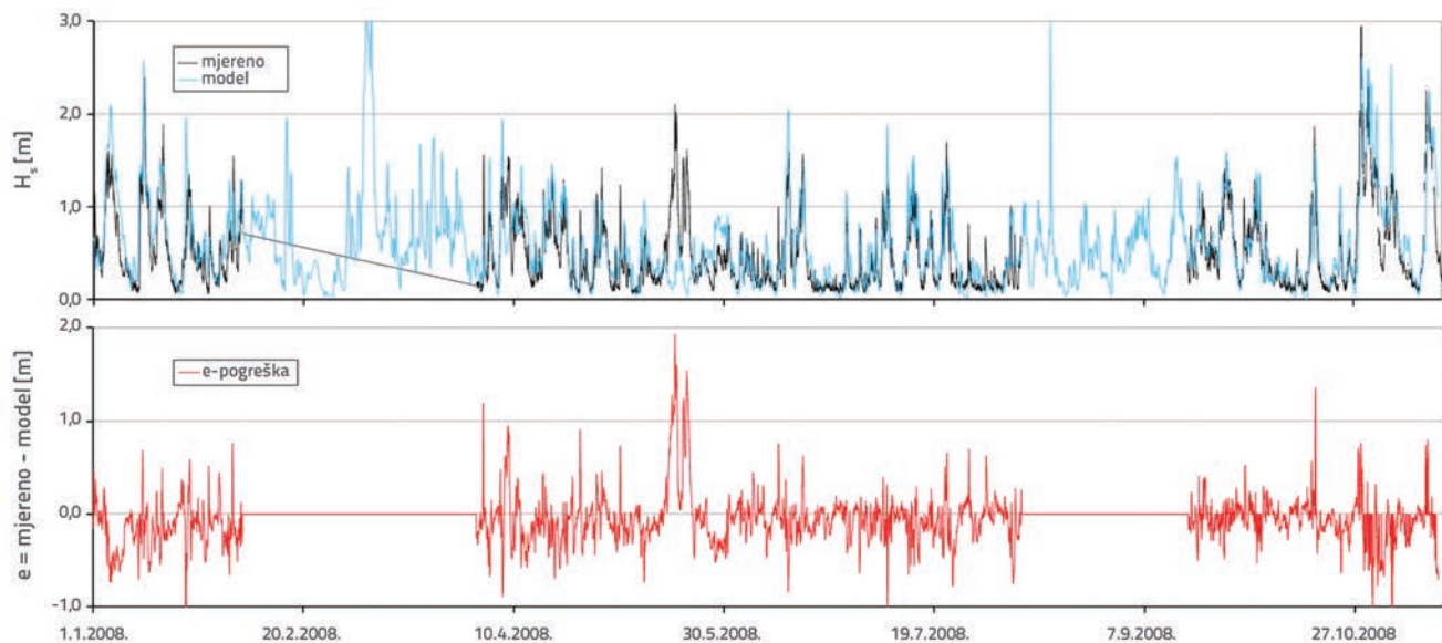
Slika 8. Usporedba izmjerene i modelirane vremenske niza značajnih valnih visina H_s na poziciji valografske postaje (gore) i histogram pogreške ( e = \text{mjereno} - \text{model} ) modelskih vrijednosti H_s za provedenu numeričku simulaciju u 2008. godini
