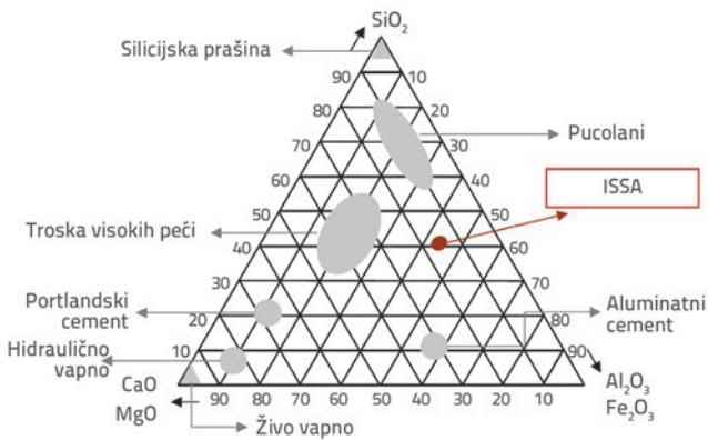
Slika 5. Trojni Keil-Rankinov dijagram za sustav \text{CaO-SiO}_2\text{-Al}_2\text{O}_3 s naznačenim položajem različitih mineralnih dodataka cementu i tipovima cementa, gdje je ISSA - pepeo dobiven spaljivanjem mulja s UPOV-a (engl. incinerated sewage sludge ash ) [27]
