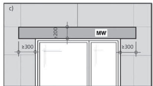
Slika 5. Protupožarna barijera: a) postavljena na uzorku EM_2; b) shema - presjek [14]; c) shema - pogled [14]
