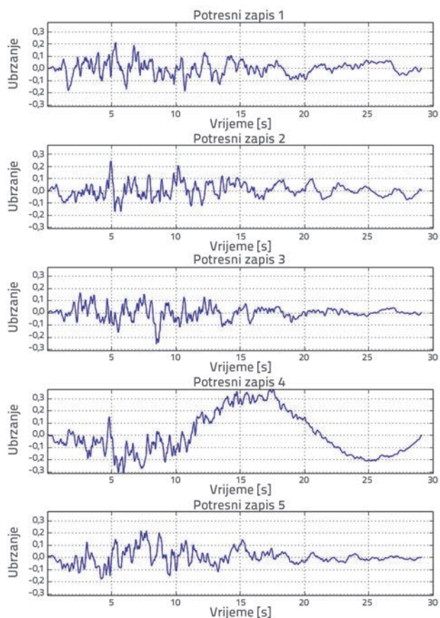
Slika 12. Umjetno generirani potresni zapisi
