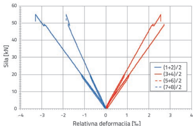
Slika 12. Dijagram sila – relativna deformacija, uzorak GR1 (mjerna mjesta: 1 i 2 gornja zona - polje, 3 i 4 donja zona - polje, gornja zona - ležaj 5 i 6 te donja zona - ležaj 7 i 8)
