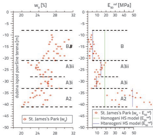
Slika 7. Određivanje računskih modula krutosti, E_{50}^{ref} homogenog i heterogenog HS modela iz korelacija s izmjerenom prirodnom vlažnosti na lokaciji St James's Park [16]
