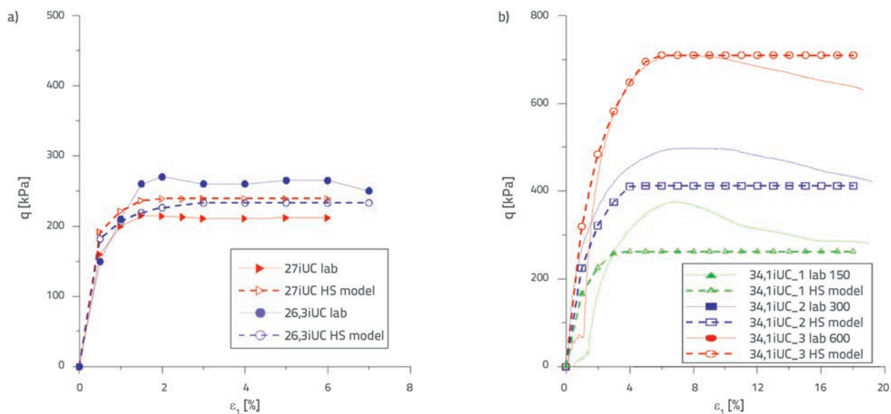
Slika 3. Simulacija troosnih nedreniranih pokusa londonske i zagrebačke gline u HS modelu: a) krivulja \varepsilon_1 - q za londonsku glinu; b) krivulja \varepsilon_1 - q za zagrebačku glinu
