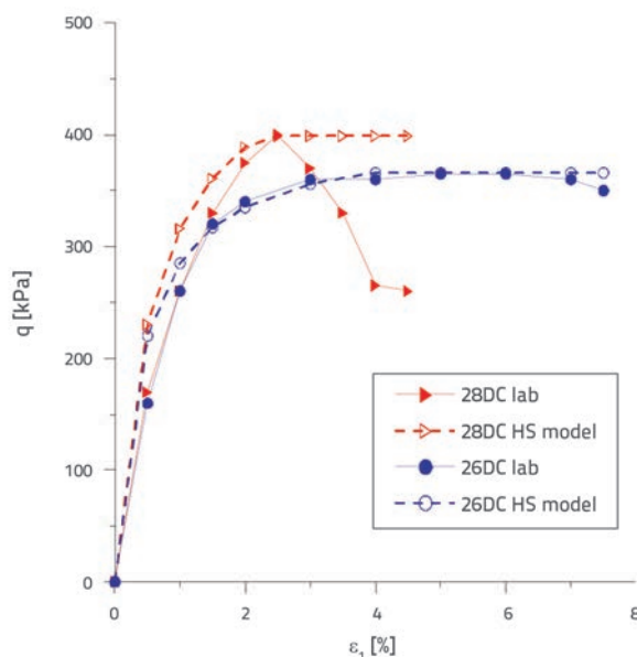
Slika 1. Simulacija troosnih dreniranih pokusa londonske gline u HS modelu, krivulja \varepsilon_1 - q
