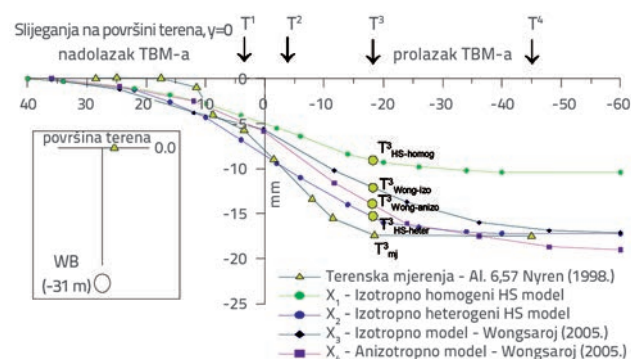
Slika 9. Postupak za utvrđivanje odstupanja između proračunanih i mjerenih slijeganja pri izgradnji zapadne tunske cijevi na lokaciji St James Park
