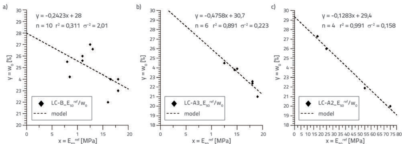
Slika 5. Lokalna korelacija E_{50}^{ref} i w_0 : a) za podsloj B londonske gline b) za podsloj A3 londonske gline c) za podsloj A2 londonske gline
