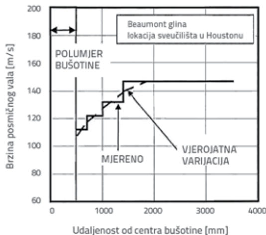
Slika 3. Utjecaj iskopa bušotine na posmični modul pri malim deformacijama za bušene pilote na lokaciji Sveučilišta u Houstonu (prekonsolidirana gлина) [6]
