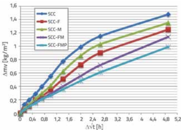
Slika 4. Grafički prikaz kapilarnog upijanja pri starosti 90 dana
