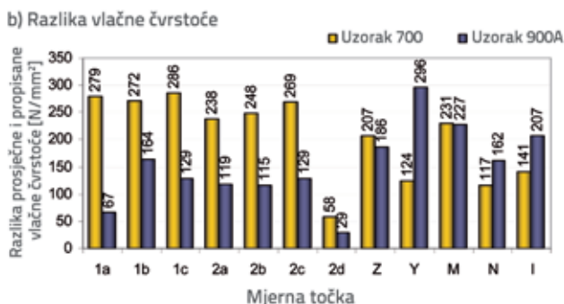
Slika 17. Razlika između proračunatih prosječnih i najmanjih propisanih vrijednosti tvrdoće i vlačne čvrstoće
