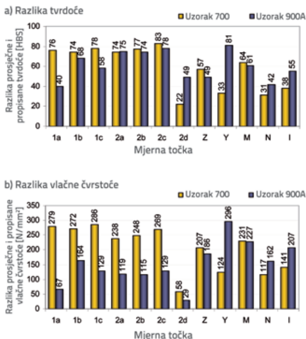
Slika 17. Razlika između proračunanih prosječnih i najmanjih propisanih vrijednosti tvrdoće i vlačne čvrstoće
