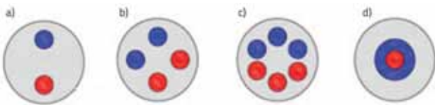
Slika 8. Raspored cijevi unutar bušotine: a) jednostruka U cijev; b) dvostruka U cijev; c) trostruka U cijev; d) koaksijalna cijev
