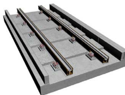
Slika 23. Konstrukcija tramvajskog kolosijeka u Zagrebu
