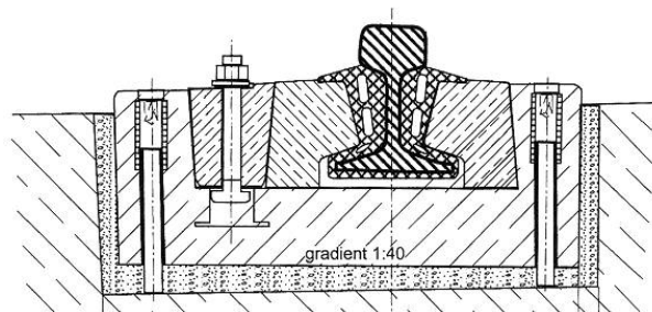
Slika 22. Poprečni presjek kolosiječnog sustava „SFF“ [1]
