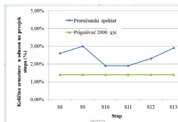
Slika 17. Količina (%) armature u stupovima za neprigušenu i prigušenu konstrukciju
