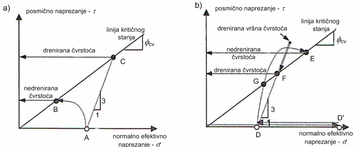
Slika 5. Drenirana i nedrenirana čvrstoća gline prema Michellu [8]: a) meke gline, b) krute gline
