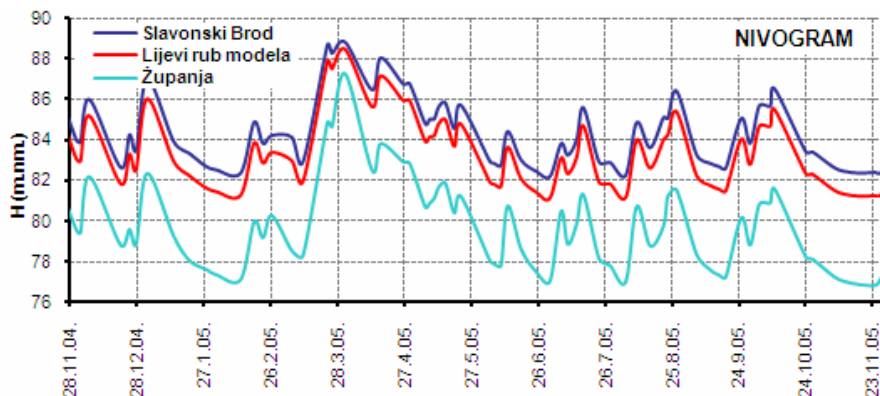
Slika 5. Nivogram Save na postajama Slavonski Brod i Županja tijekom razdoblja 28.11.04. do 28.11.05. i usvojeni nivogram Save na lokaciji lijevog ruba modeliranog područja
