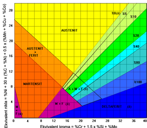
Slika 2. Schaeffleov dijagram podjele nehrđajućih čelika [8]
