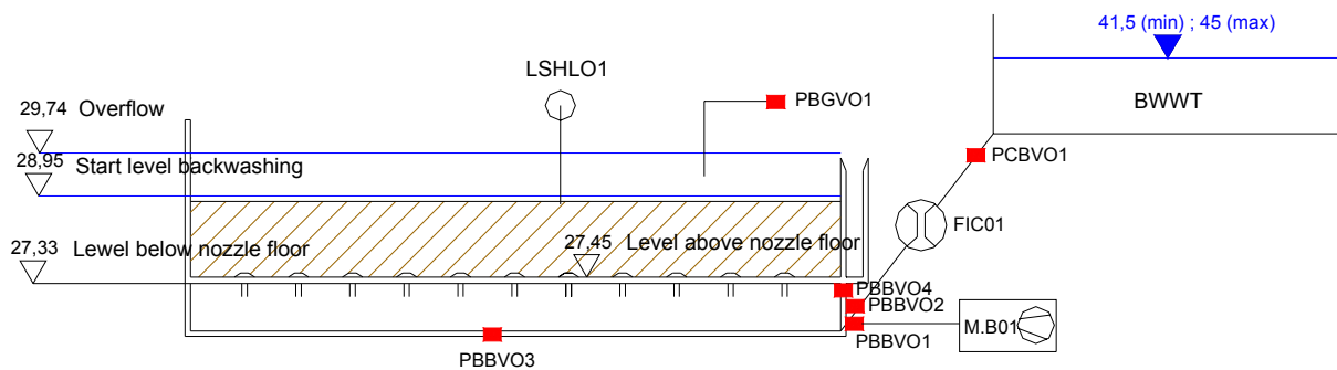
Slika 1. Shematski prikaz glavnih građevinskih i hidrauličkih dijelova vezanih za proces ispiranje brzih filtera u Tvornici vode «Butoniga»
