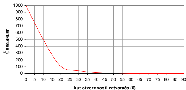
Slika 5. Krivulja koeficijena lokalnog gubitka za «butterfly» ventile PCBV01 i PBBV02
