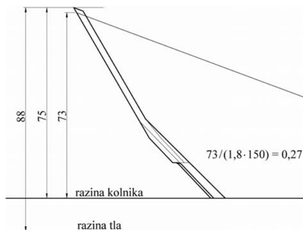
Slika 14. Određivanje visine pilona mosta Jarun
