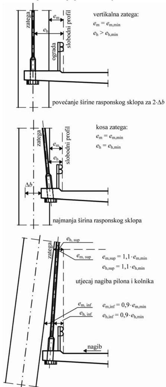
Slika 15. Slobodan prostor potreban kod ovješnja u dvije ravnine
