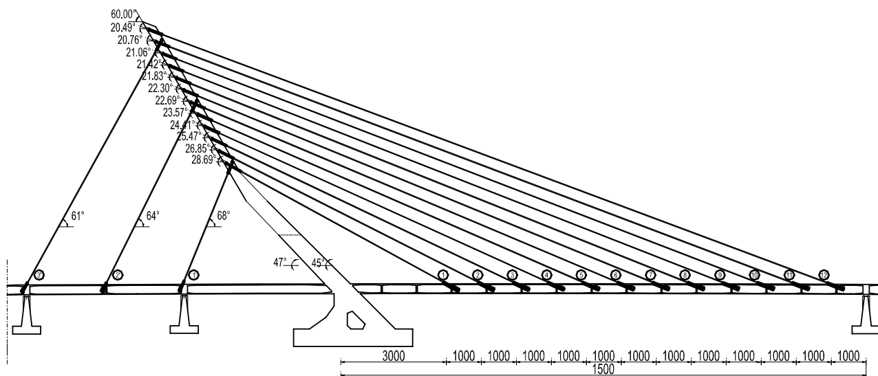
Slika 13. Raspored zatega mosta Jarun
