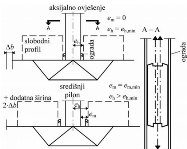
Slika 16. Slobodan prostor potreban kod ovješnja u jednoj ravlini
