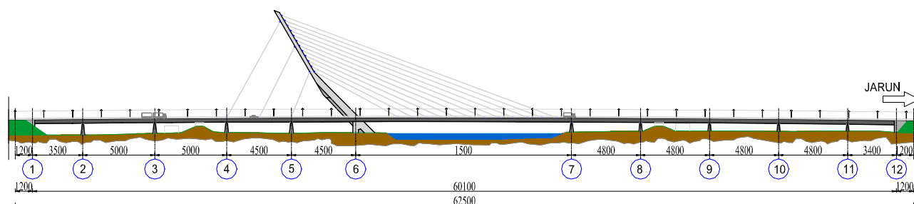
Slika 2. Uzdužni presjek mosta Jarun
