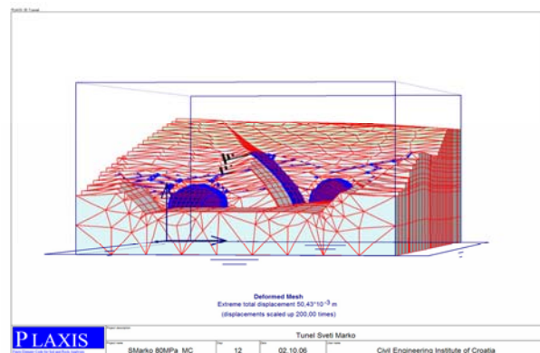
Slika 9. Geometrija numeričkog modela predusjeka tunela Sv. Marko
