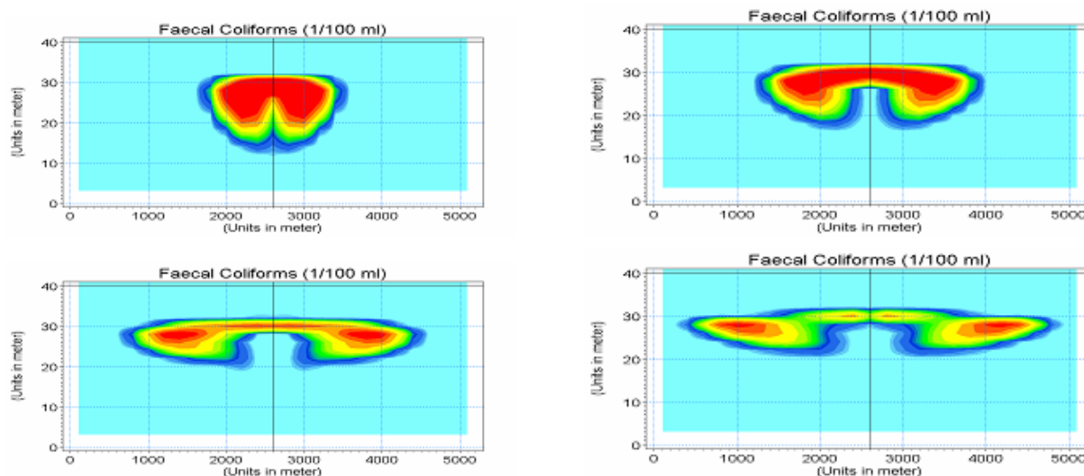
Slika 4. Prikaz koncentracije fekalnih koliforma u poprečnom presjeku na udaljenosti 1000 (lijevo gore), 2000 m (desno gore), 4000 m (lijevo dolje) i 6000 m (desno dolje) od lokacije pridnenoga ispuštanja onečišćenja (eksperiment 35/15/10_30/3D → piknoklina na 10 m dubine)
