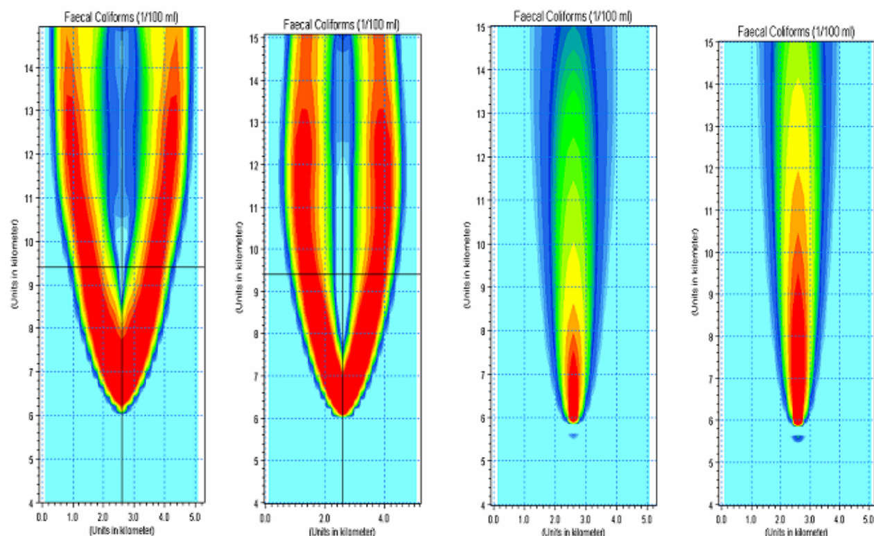
Slike 6., 7., 8. i 9. Prostorna raspodjela koncentracija fekalnih koliforma u horizontalnom sloju na dubini od 2 do 4 m ispod piknokline za 3D numeričke pokuse 3,5/15/10_30/3D (prva s lijeve strane), 3,5/15/20_20/3D (druga s lijeve strane) odnosno za 2D numeričke pokuse 3,5/15/10_30/2D (treća s lijeve strane) i 3,5/15/20_20/2D (četvrta s lijeve strane)
