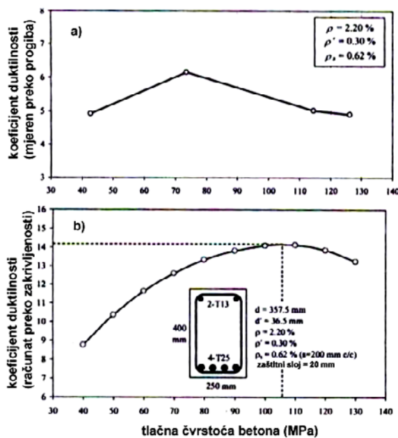
Slika 6. Duktilitet armiranobetonske grede u ovisnosti o čvrstoći betona prema eksperimentalnim (a) i analitičkim (b) rezultatima [20]
