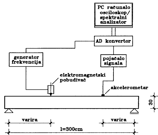
Slika 7. Shematski prikaz mjerenja vlastitih frekvencija grede
