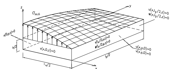
Slika 7. Rubni uvjeti i opterećenje za osminu ploče
