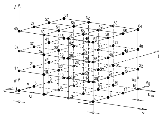
Slika 5. Konačni element u obliku kvadra sa 64 čvora
