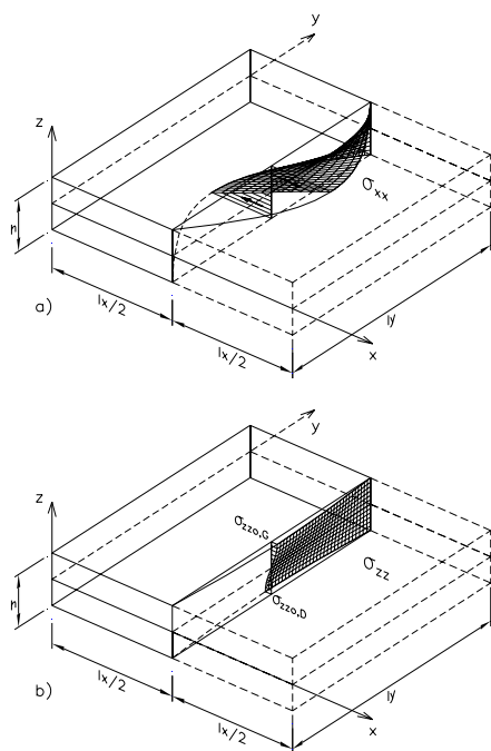
Slika 3. Normalna naprezanja u ravnnini x = l_x/2 : a) \sigma_{xx} , b) \sigma_{zz}
