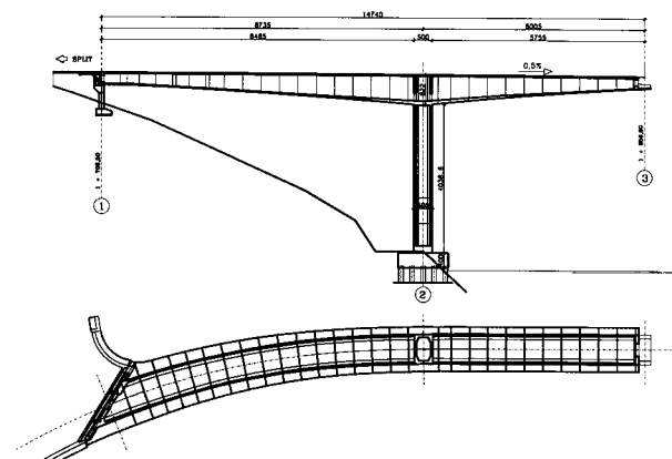
Slika 13. Uzdužni presjek i tlocrt prednapetog betonskog mosta
