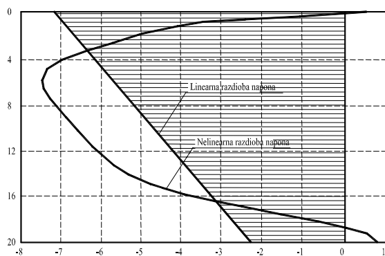
Slika 9. Razdioba naprezanja na ploči debljine 20 cm opterećene ekscentričnim tlakom, t = 28 dana
