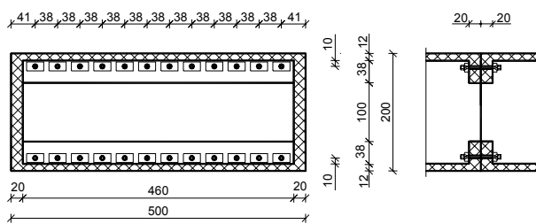
Slika 10. Raspored prednapetih šipki \phi 36 mm na spojevima odsječaka stupa
