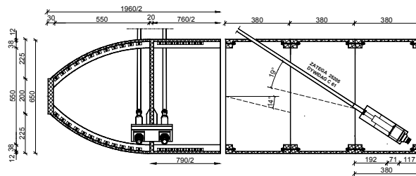
Slika 13. Sidrenje vješaljki u luku i spajanje odsječaka prednapetim šipkama \phi 36 mm
