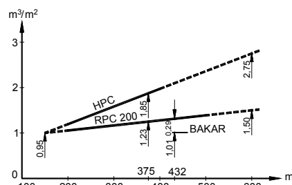
Slika 16. Dijagrami količina betona po m^2 tlocrta
