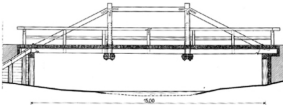
Slika 2. Tipski drveni cestovni most raspo na 15 m, Ministarstvo građevina Kraljevine Jugoslavije, 1929.
