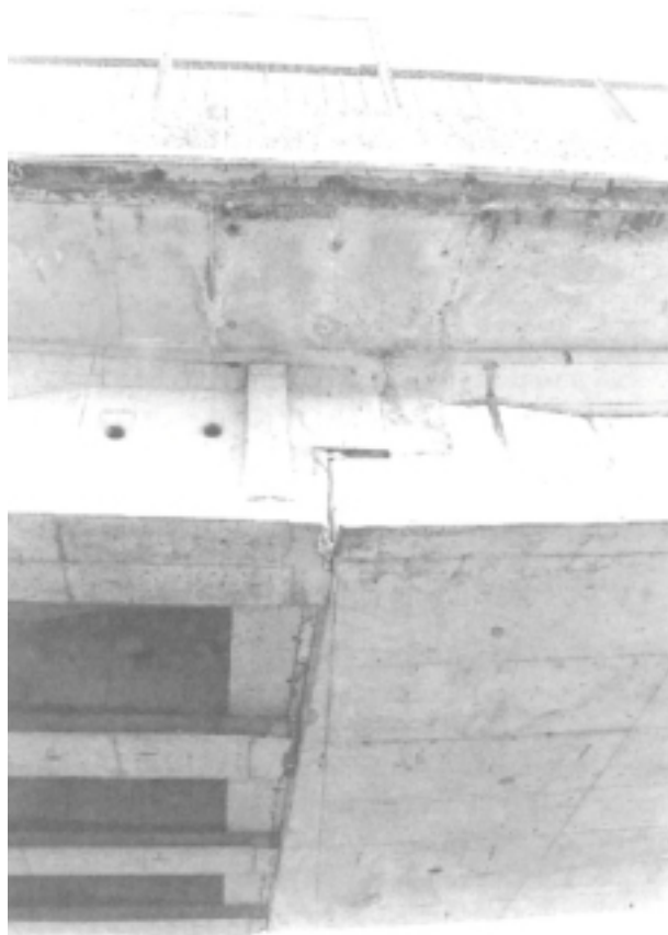
Slika 4. Neuređan detalj oslanjanja prednapetoga roštiljnog sklopa na proširenu naglavnicu
