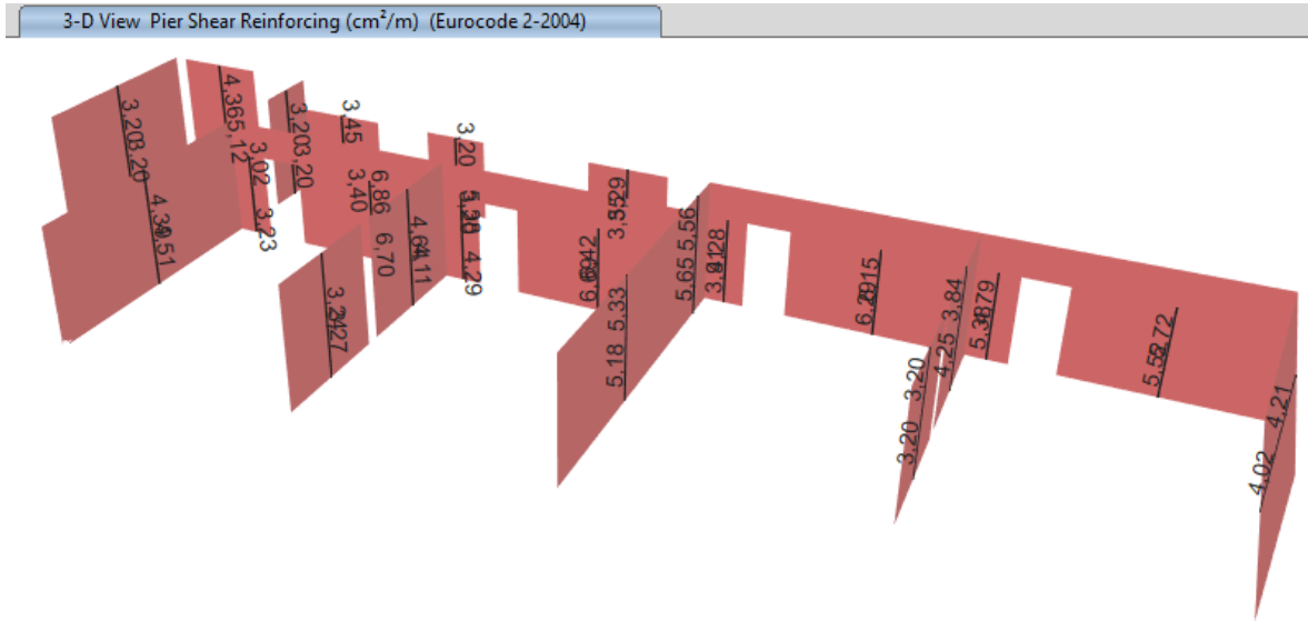
Slika 167: Potrebne količine horizontalne armature u zidovima prema mjerodavnoj kombinaciji PTRRSQ [cm²/m]
