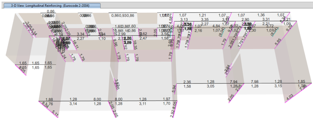
Slika 168: Potrebne količine uzdužne armature u stupovima i horizontalnim serklažima prema mjerodavnoj kombinaciji PTRRSQ [cm²]
