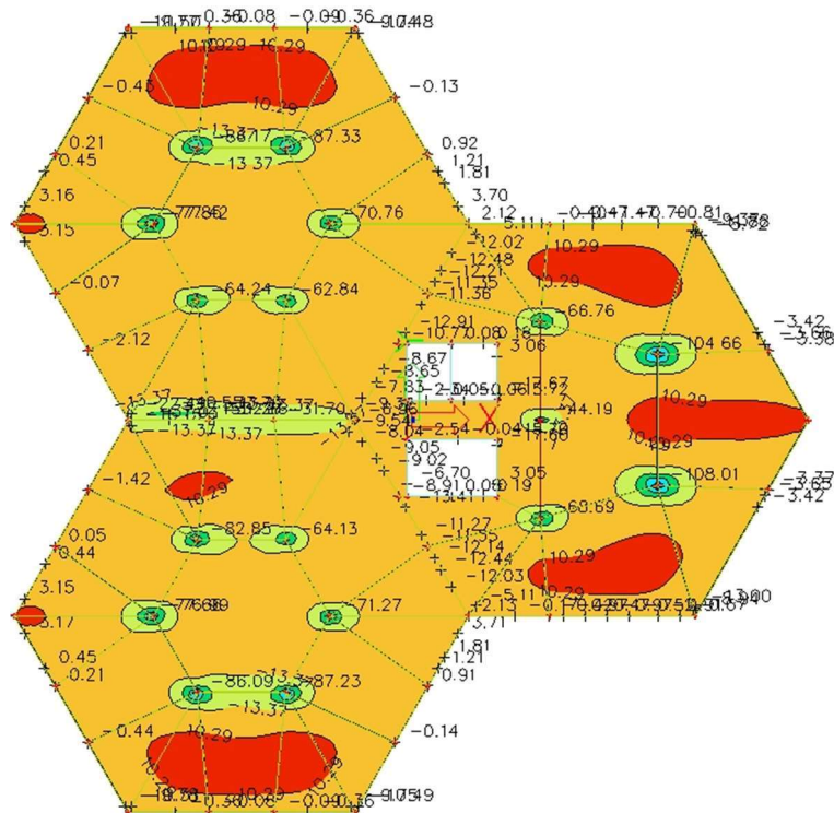
Slika 75.: Anelopa maksimalnih momenata savijanja u Y smjeru (GSN) – ležaj
