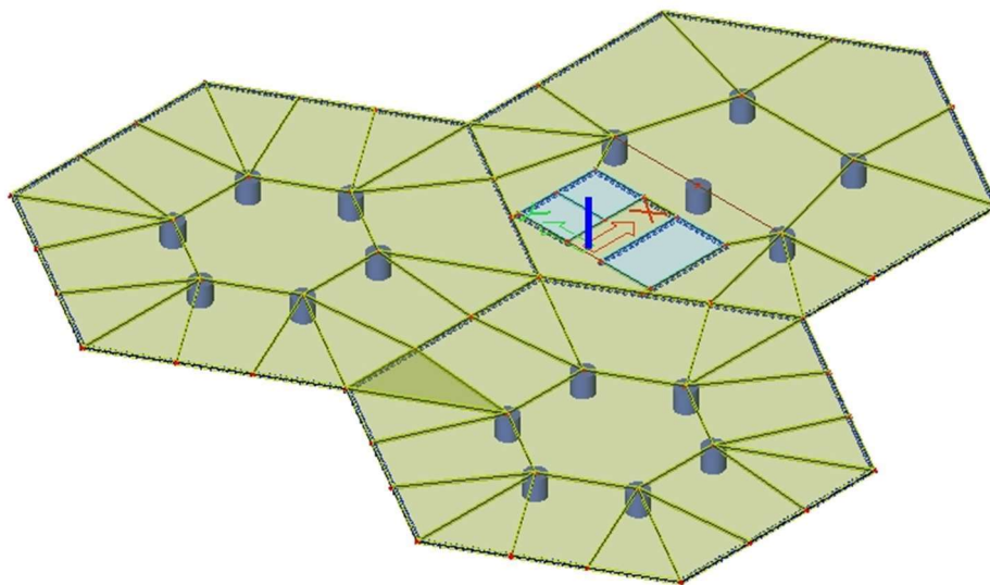
Slika 97.: Prikaz lokalnog modela ploče u programu SCIA Engineer
