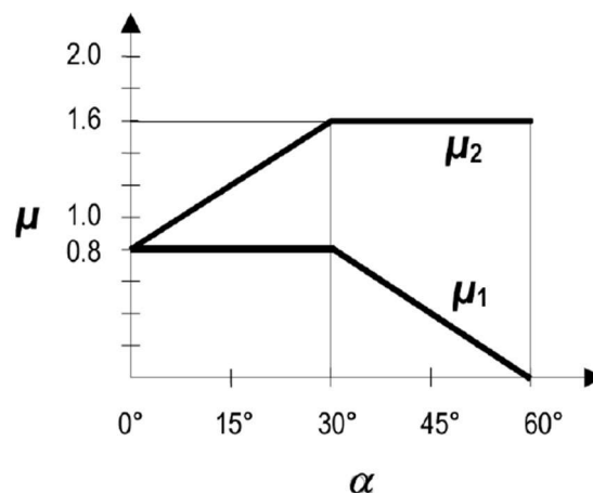
Slika 10.: Koeficijenti oblika opterećenja snijegom (Izvor: [5])
