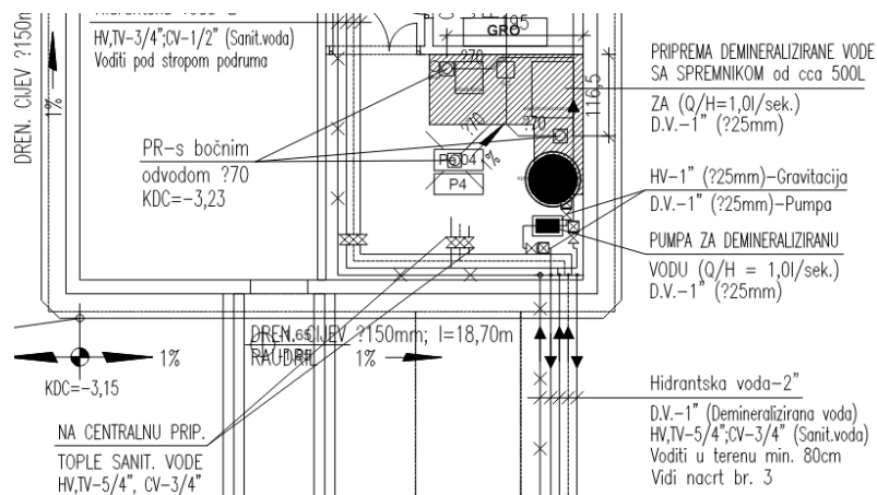
Slika 26.: Tehnički prikaz vodovodnih i kanalizacijskih instalacija (Izvor: [29])
