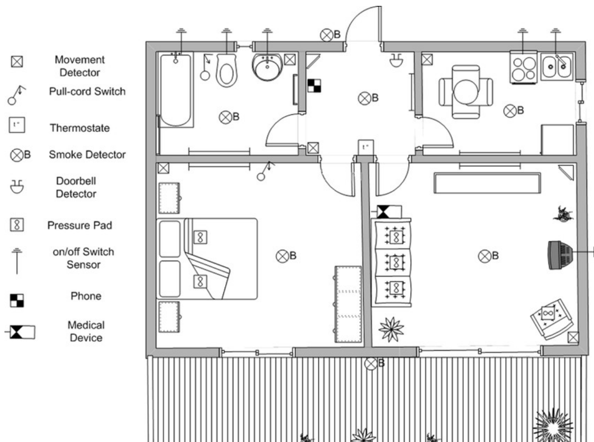
Slika 16.: Tlocrt pametne kuće (Izvor: [22])
