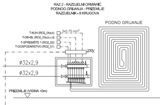
Slika 27.: Prikaz podnog grijanja (Izvor: [30])
