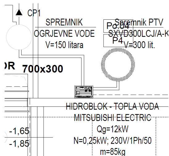
Slika 22.: Komponente sustava za pripremu sanitarne tople vode (Izvor: [25])
