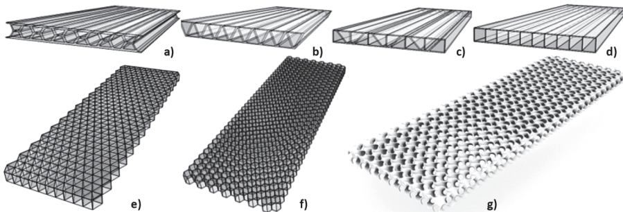
Slika 3. FRP ploče, primjer adhezivno spojenih vučenih profila: a) Superdeck; b) EZSpan; c) DuraSpan; d) Strongwell - Primjeri sendvič-panela s: e) trokutastom ispunom; f) sačastom ispunom i primjeri trodimenzionalne ispune: g) Gyroid
