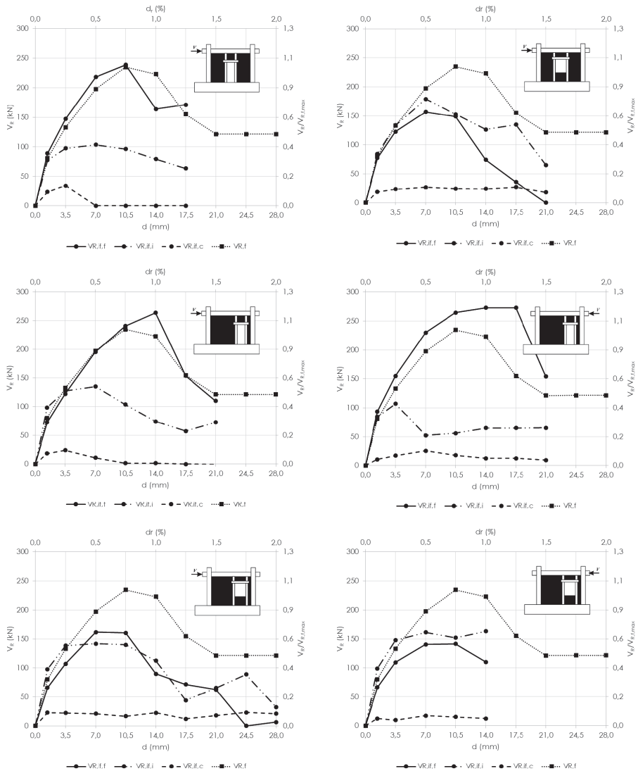
Slika 6. Razdioba posmične otpornosti na elemente konstrukcijskoga sustava okvir-zid (Skupina II)
