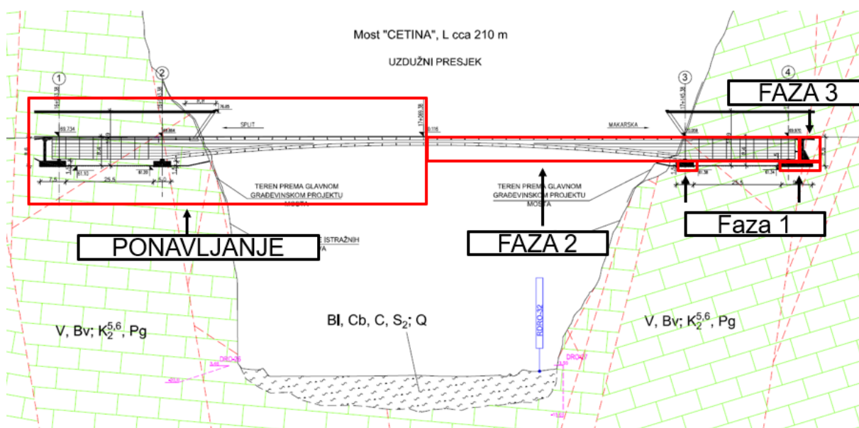
Slika 20.: Uzdužni presjek mosta, sa fazama gradnje mosta
