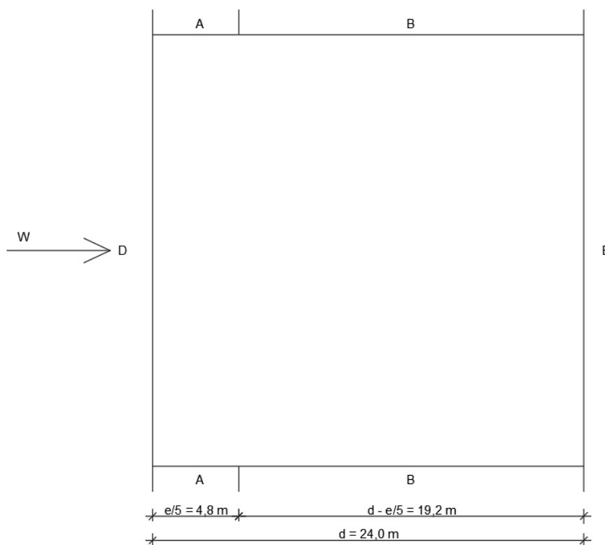
Slika 2.5 Podjela vertikalnih površina u tlocrtu
