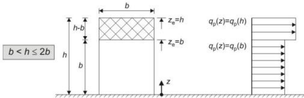
Slika 2.2 Raspodjela tlaka vjetra po visini (Izvor: [13])
