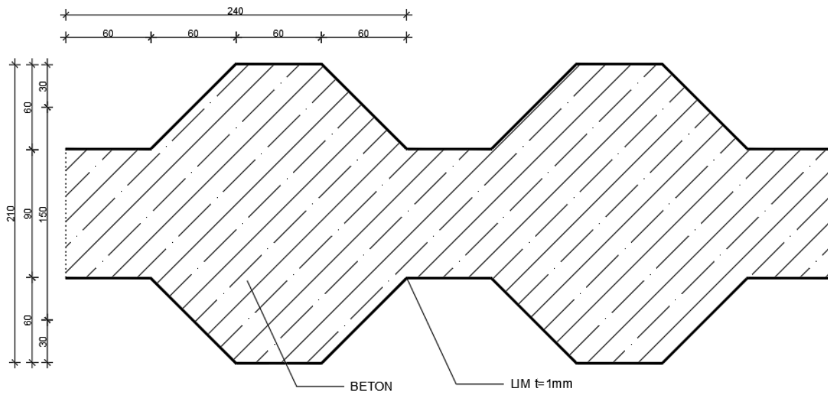
Slika 5.1 Poprečni presjek posmičnog zida
