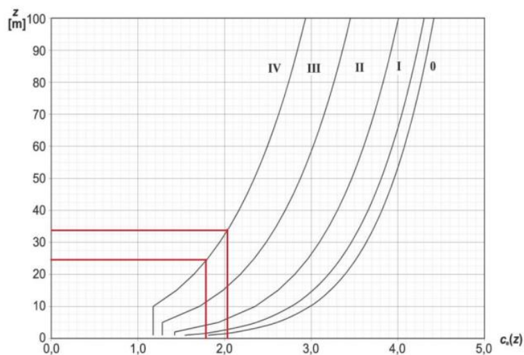
Slika 2.3 Grafički prikaz faktora izloženosti c_e(z) za c_0=1,0 , k_t=1,0 (Izvor: [13])
