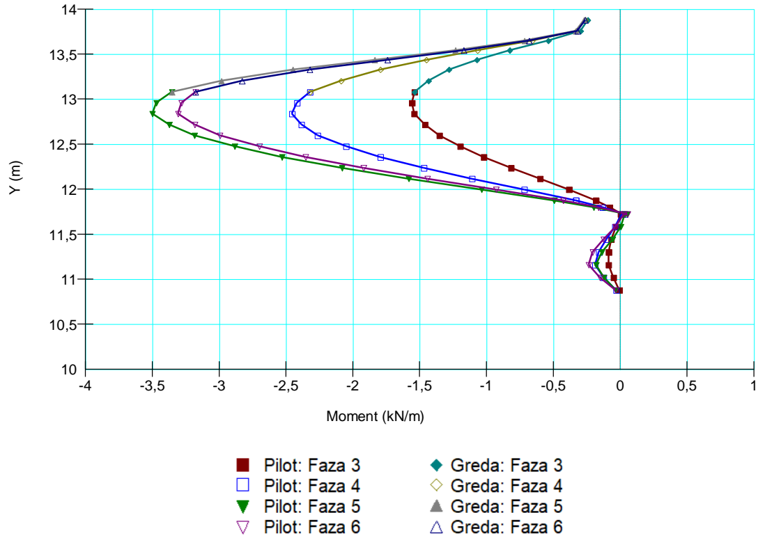
Slika 71.: Graf momenta pilotne stijene
