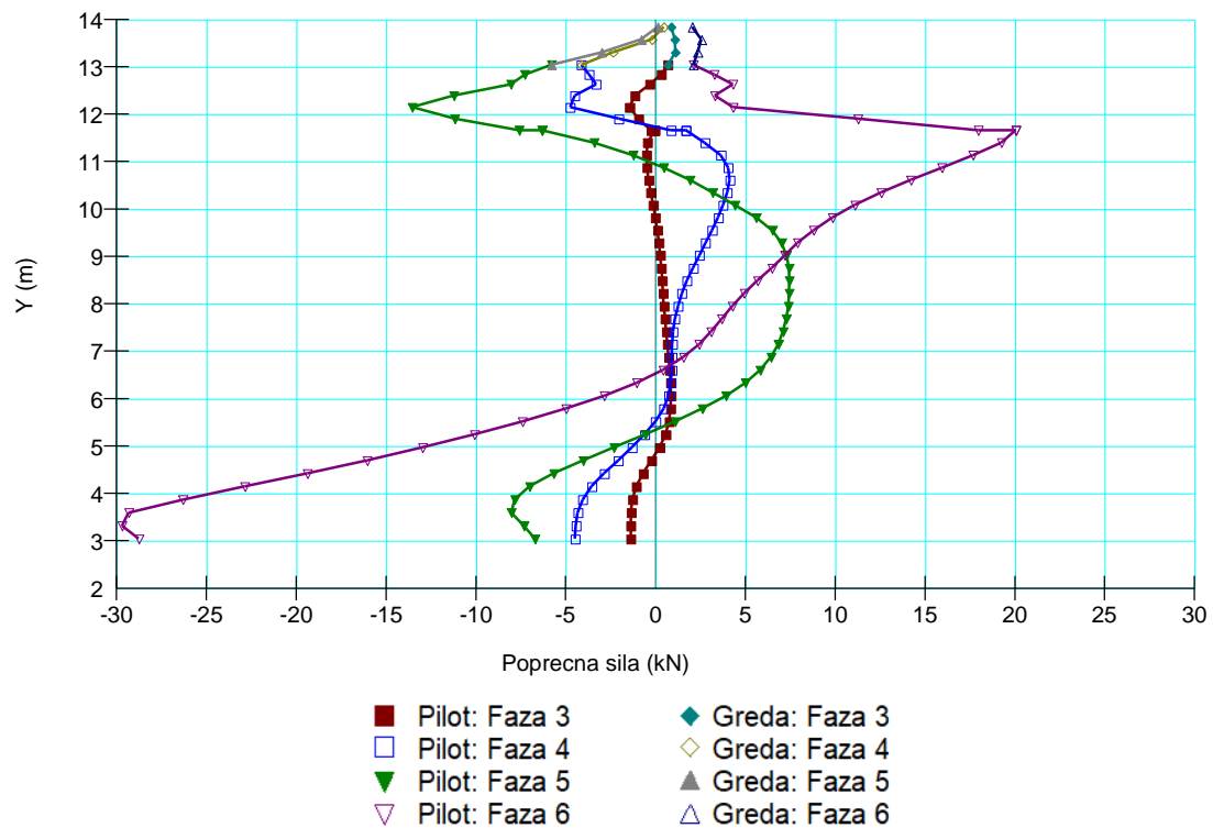
Slika 90.: Graf poprečnih sila pilotne stijene
