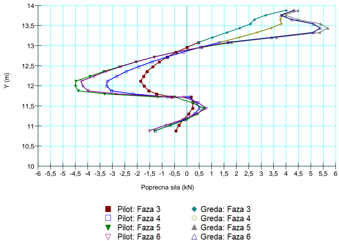
Slika 72.: Graf poprečnih sila pilotne stijene
