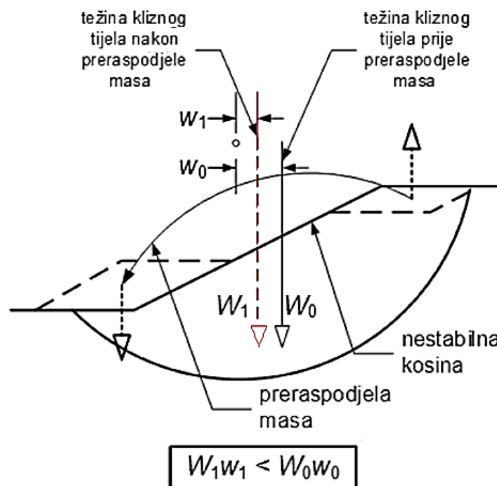
Slika 6.: Shematski prikaz preraspodjele mase kosine (Izvor: [1])
