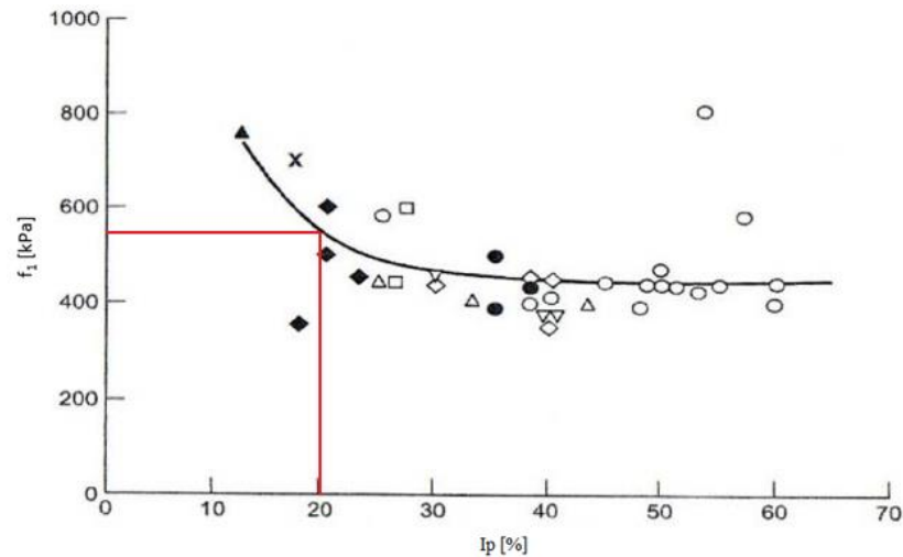
Slika 35.: Dijagram ovisnosti koeficijenta f_2 u odnosu na indeks plastičnosti (Izvor: [8])
