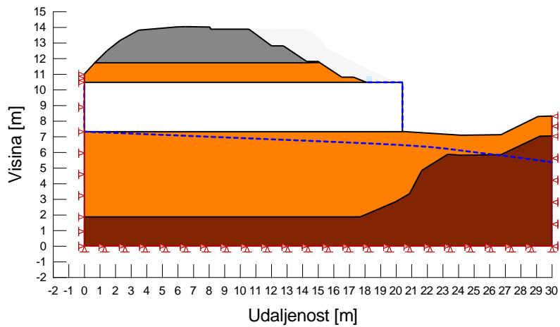
Slika 66.: Faza 2-stanje napreznja prilikom iskopa
