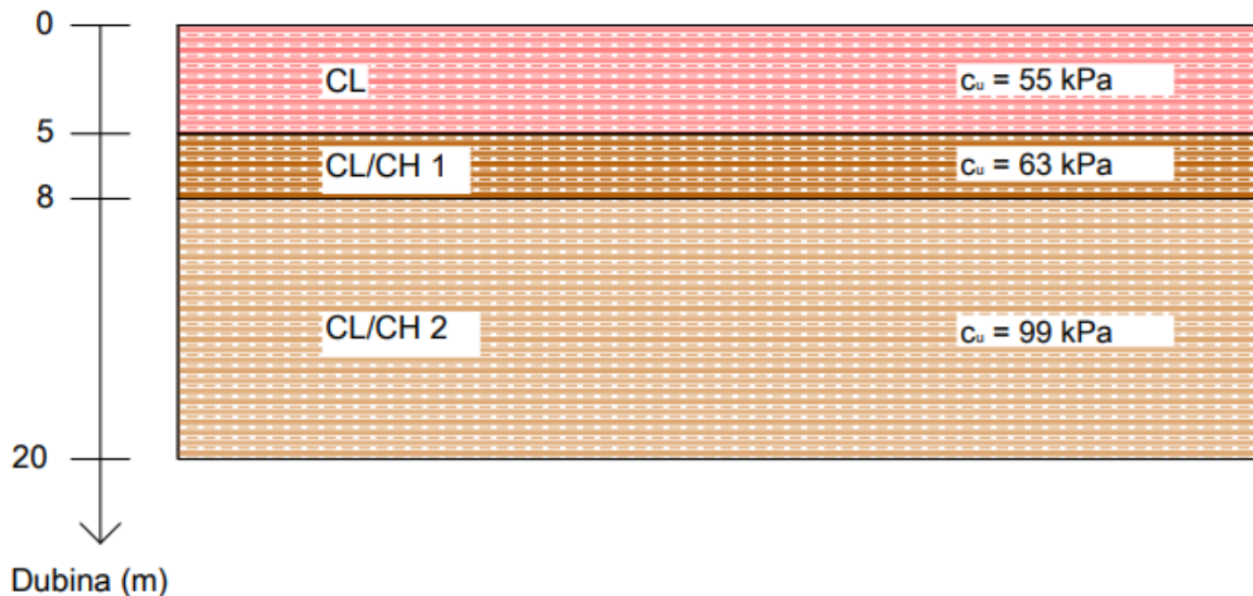
Slika 21.: Geotehnički profil tla
