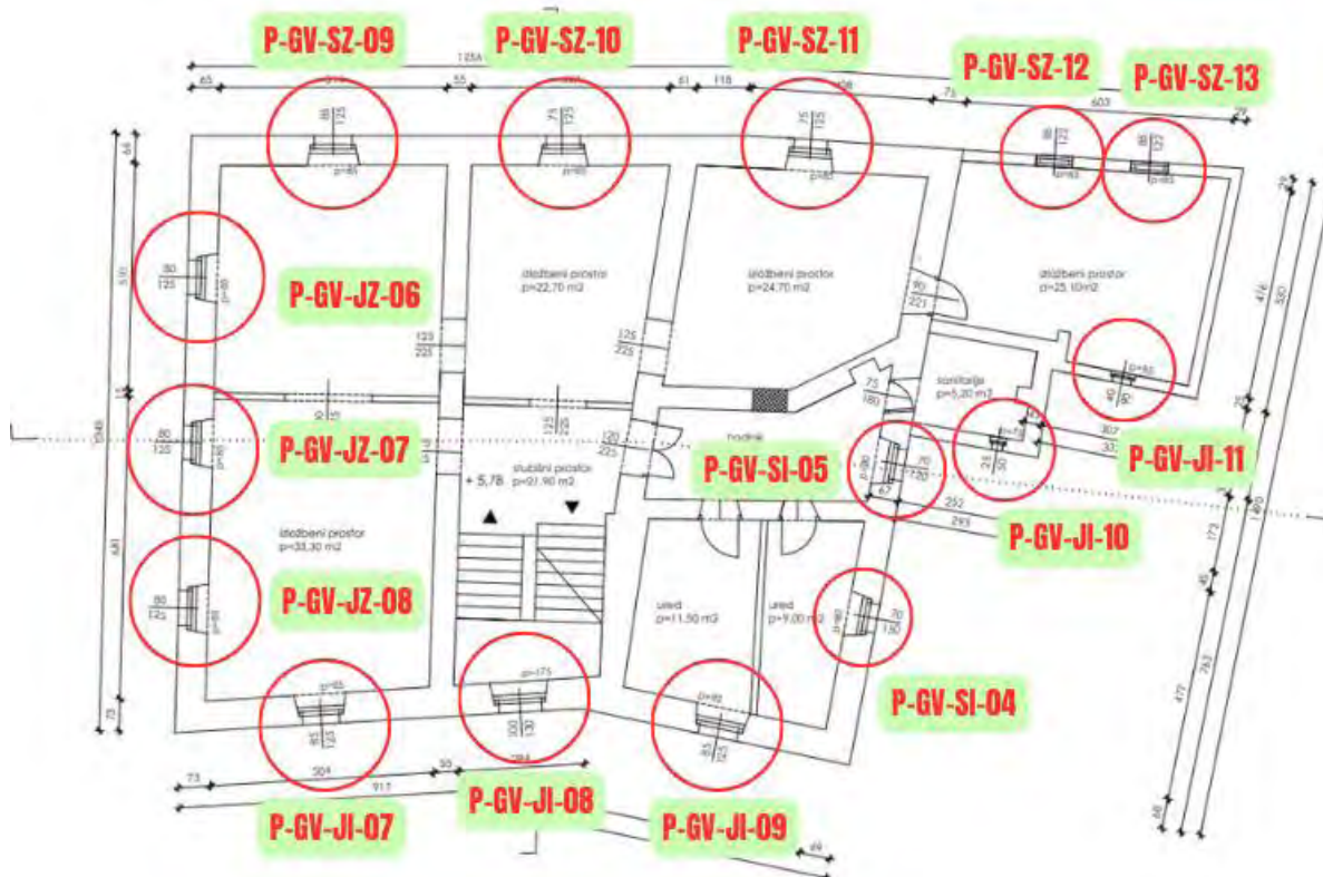
Slika 18. Raspored otvora na drugom katu
