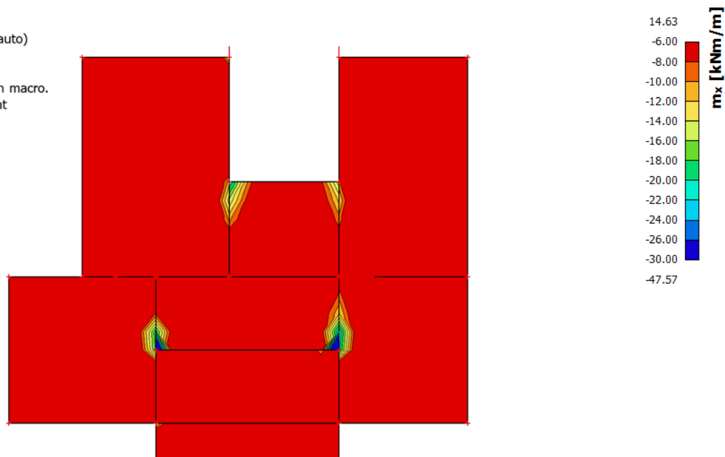
Slika 24: Momenti u x smjeru manji od srednjeg negativnog momenta
