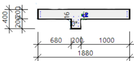
Slika 42: Poprečni presjek grede B16
