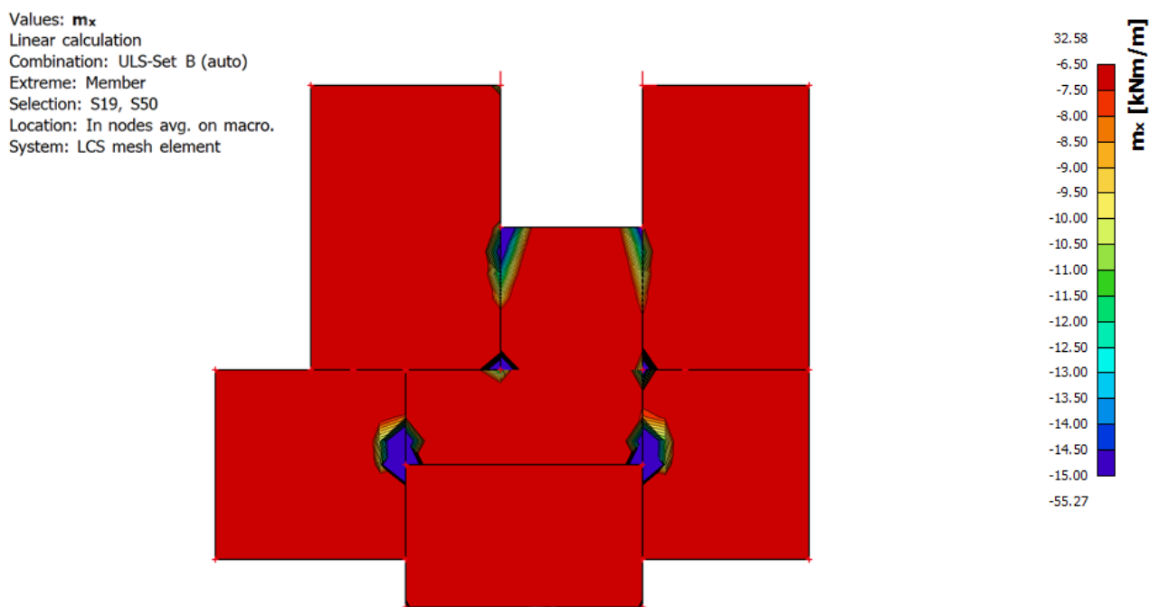
Slika 18: Momenti u x smjeru manji od srednjeg negativnog momenta
