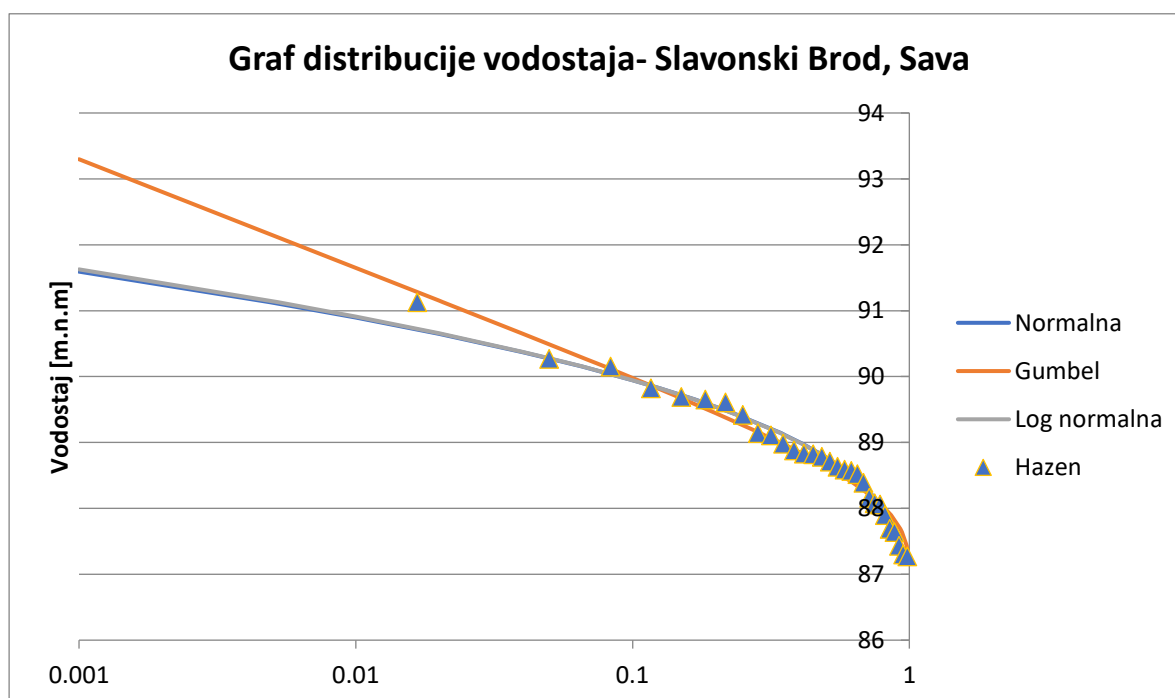
Slika 18. Rezultati teorijske vjerojatnosti pojave vodostaja, vodomjerna postaja Slavonski Brod
