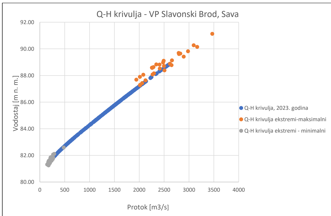
Slika 15. Konsumpcijska krivulja – vodomjerna postaja Slavonski Brod
