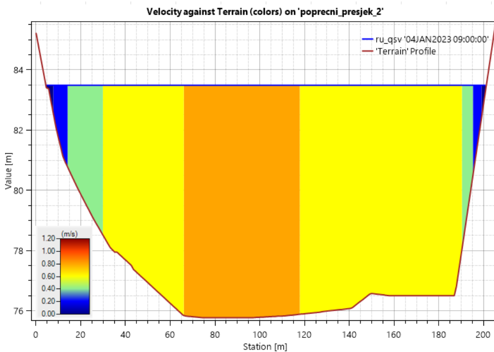
Slika 40. Raspored brzina kroz poprečni presjek 2, regulirano stanje
