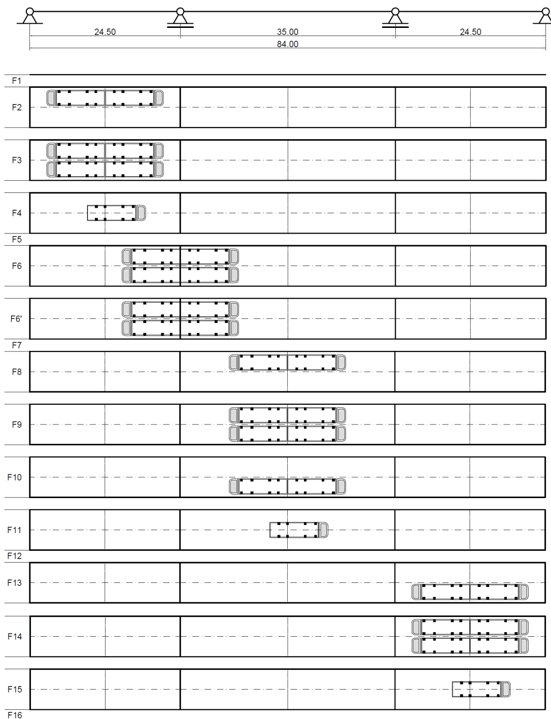
Slika 9. Shematski prikaz faza probnog opterećenja, statičko djelovanje
