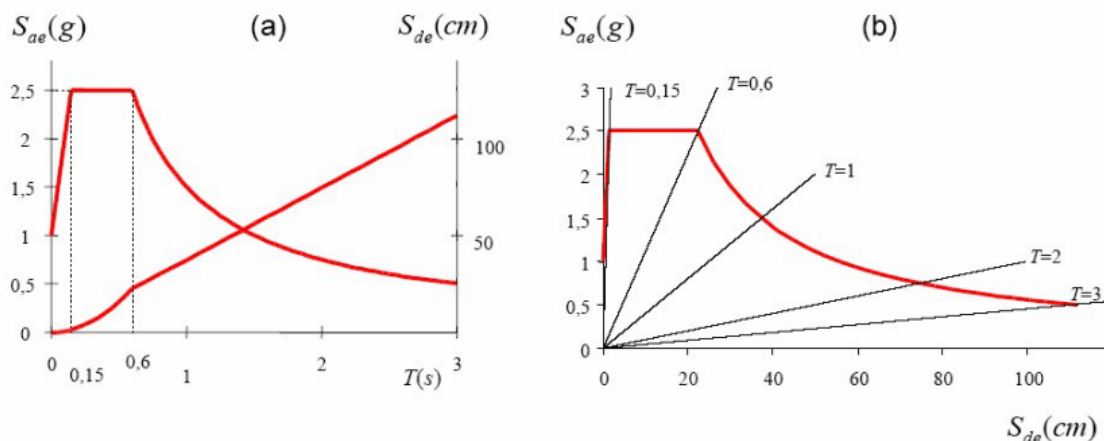
Slika 16 Elastični spektar ubrzanja i pomaka u tradicionalnom (a) i AD formatu (b) [28]
