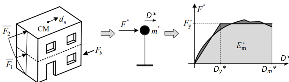
Slika 18 Svođenje na ekvivalentan jednostupanjski sustav [25]
