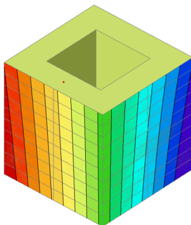
Slika 145.: Prikaz naprezanja za nazovistalnu kombinaciju djelovanja
