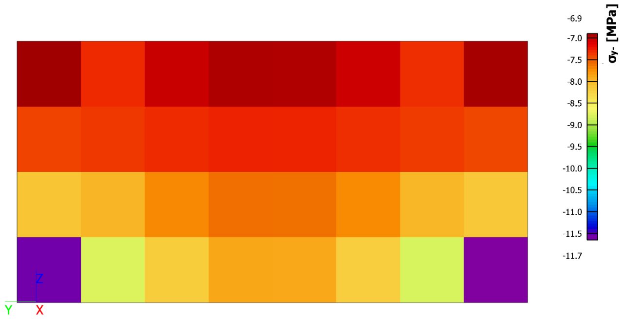
Slika 95. Grafički prikaz mjerodavnog tlačnog naprezanja za zidove jezgre d = 60 cm (karakteristična kombinacija)
