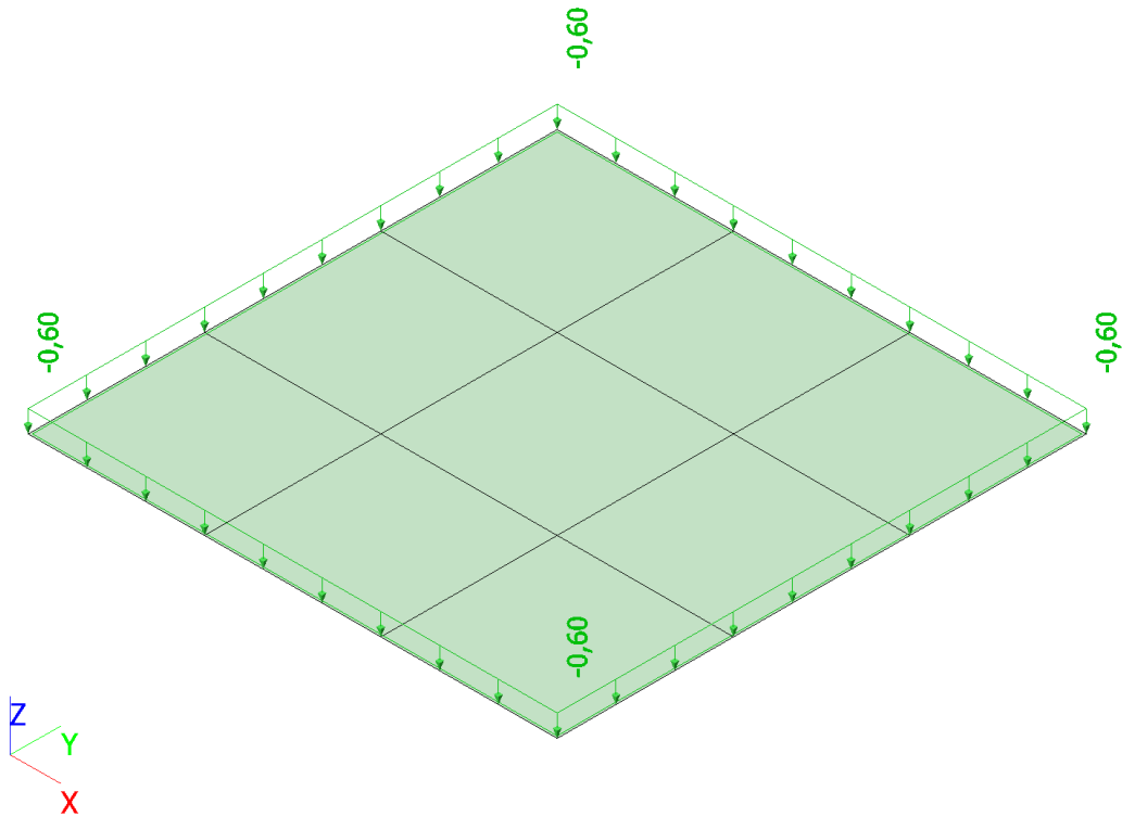
Slika 40. Uporabno opterećenje krovne konstrukcije [ \text{kN/m}^2 ]
