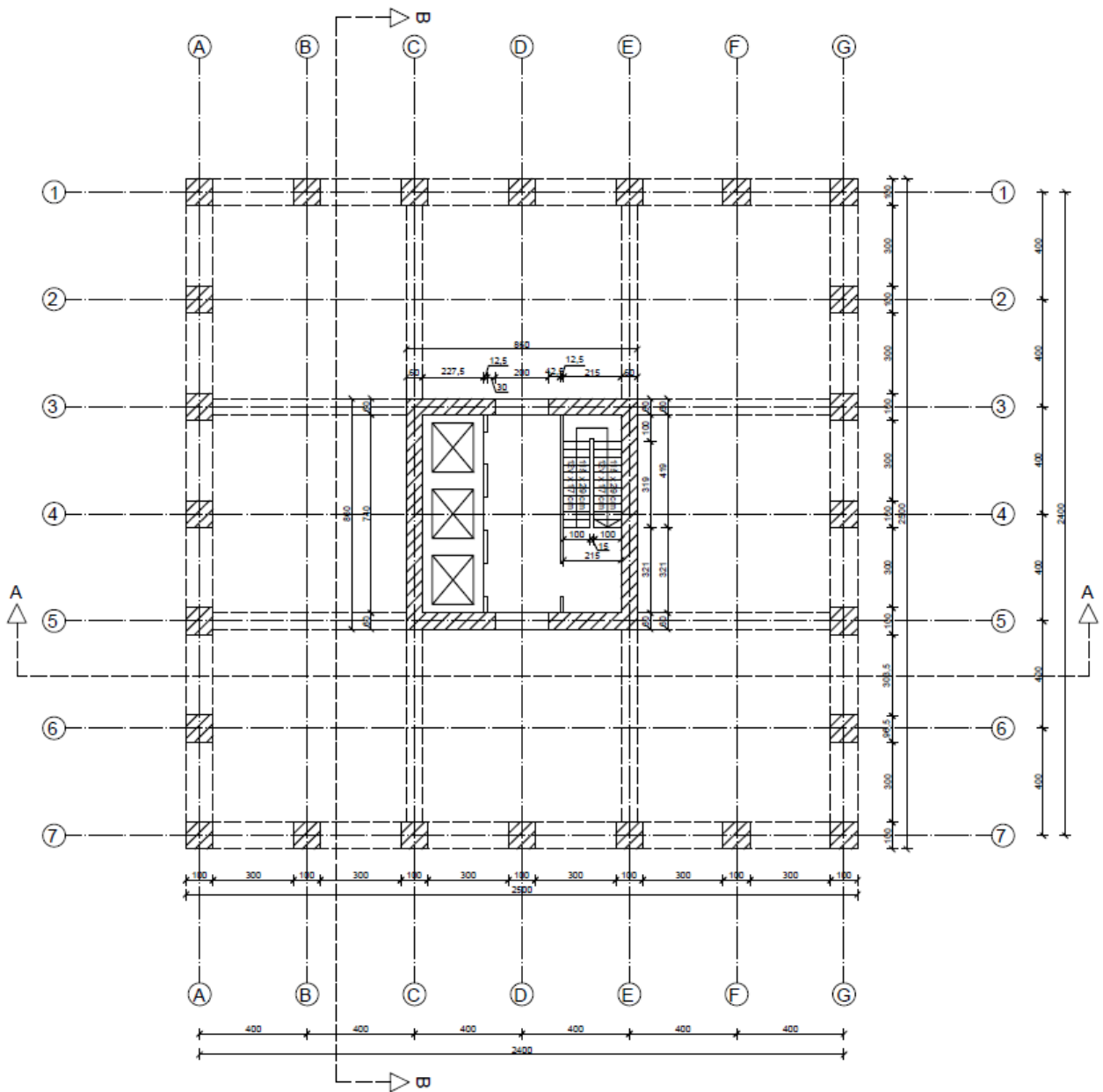
Slika 10. Tlocrt etaža 55-68
