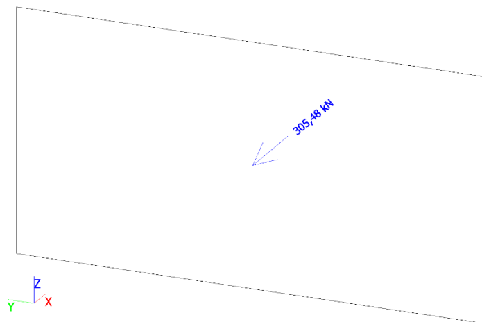
Slika 88. Grafički prikaz mjerodavne sile V_{Ed} za zidove jezgre d = 60 cm (GSN kombinacija)
