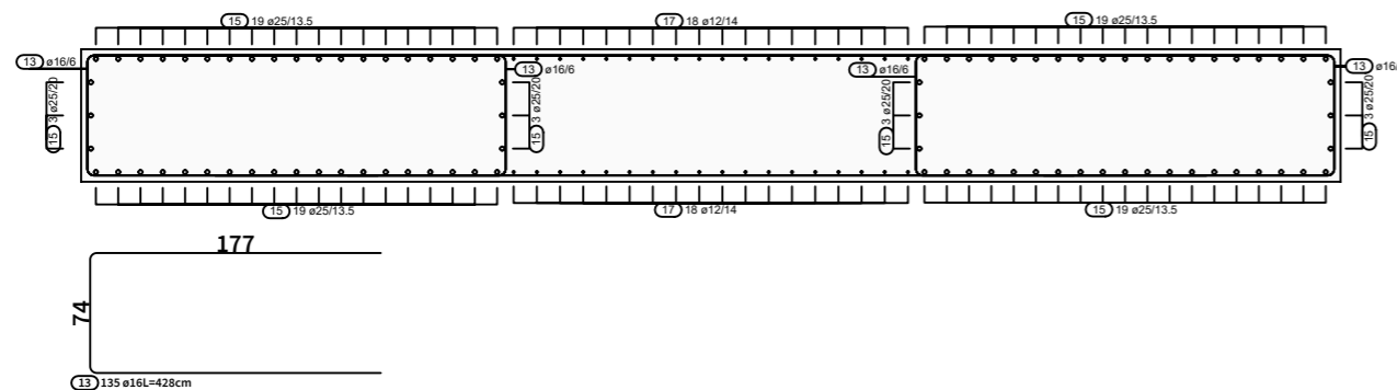
Presjek 1 - 1
