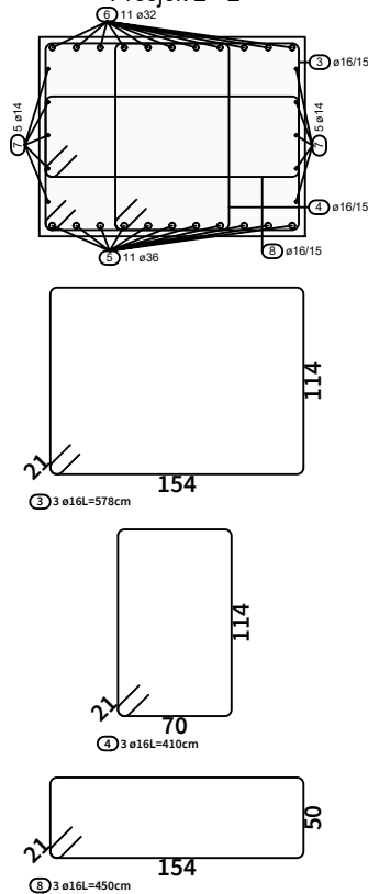
Presjek 2 - 2
