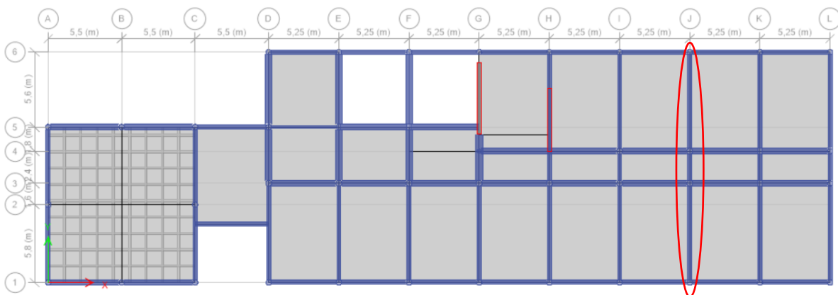
Slika 42 Prikaz izdvojenog okvira iz tlocrta prostorne konstrukcije
